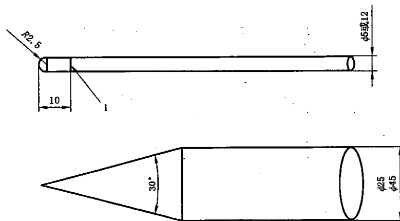
图 6 塞规
